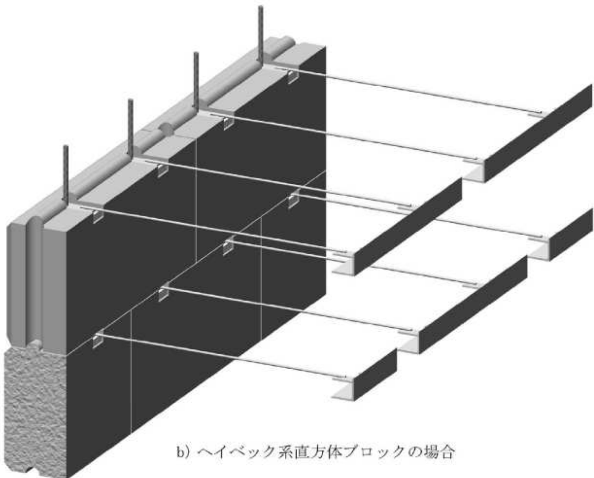
図-2.3 補強材取付部ディーテール
