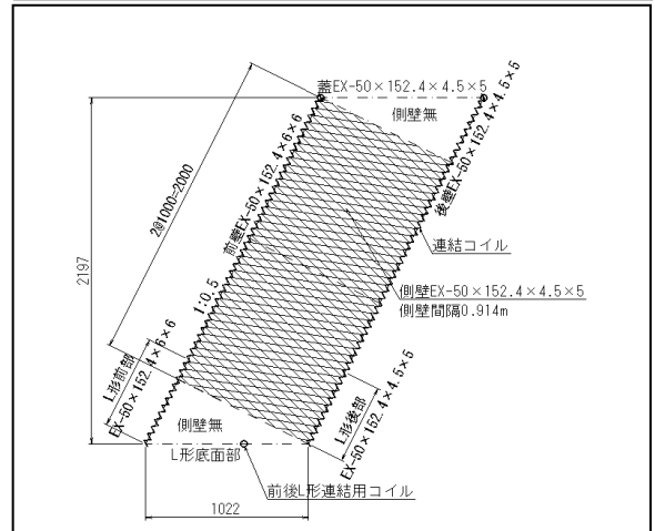
標準断面
